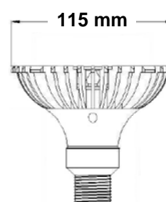
PAR36
