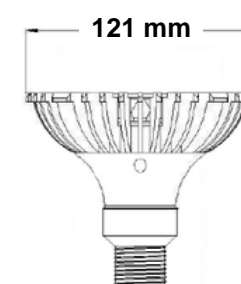
PAR38
