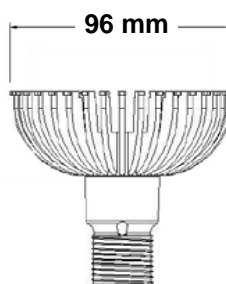
PAR30
